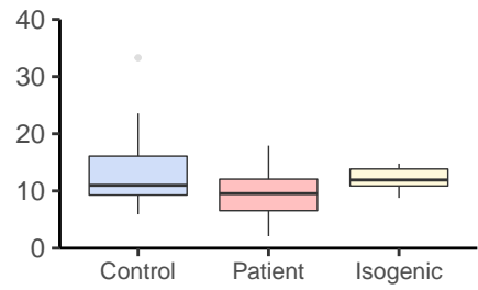
ATP.Production
